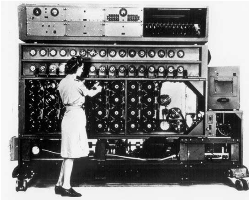
Slika 4. BOMBA, uređaj za dekriptiranje ENIGME - Encyclopedia Britannica
