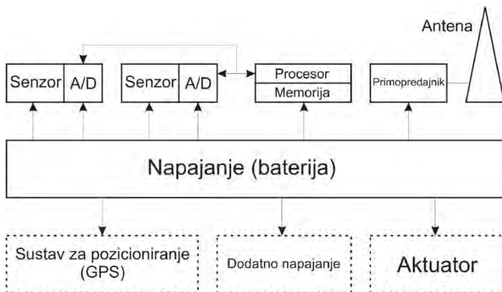
Slika 4. Struktura bežičnog senzorskog čvora (Grgić, 2011)
